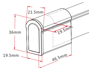
END CAP
